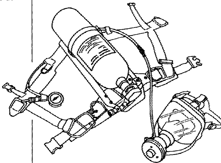
Ejemplar de un aparato independiente de respiración (SCBA), MSHA/NIOSH tipo TC-13F.
